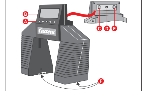
1 Elektronischer Rundenzähler
